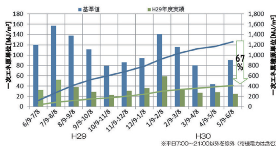
図4 一次エネルギー原単位の推移&lt;事例1&gt;
