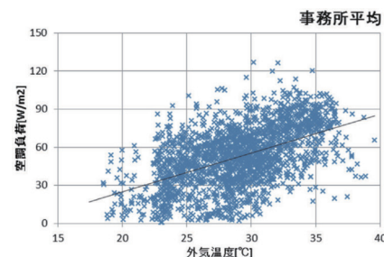
図2 空調運転データの分析(更新前)&lt;事例1&gt;
