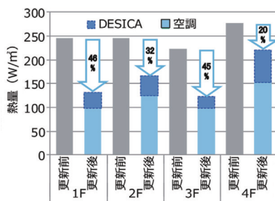
図3 空調機器の選定&lt;事例1&gt;
